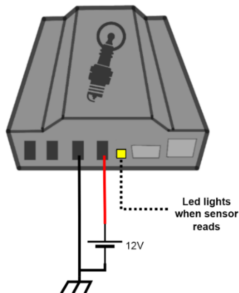
Figure 8: connessione per uso del led
